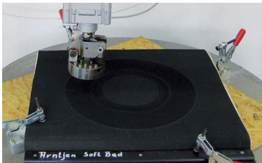
Bild 4: Dauertrittbelastung
