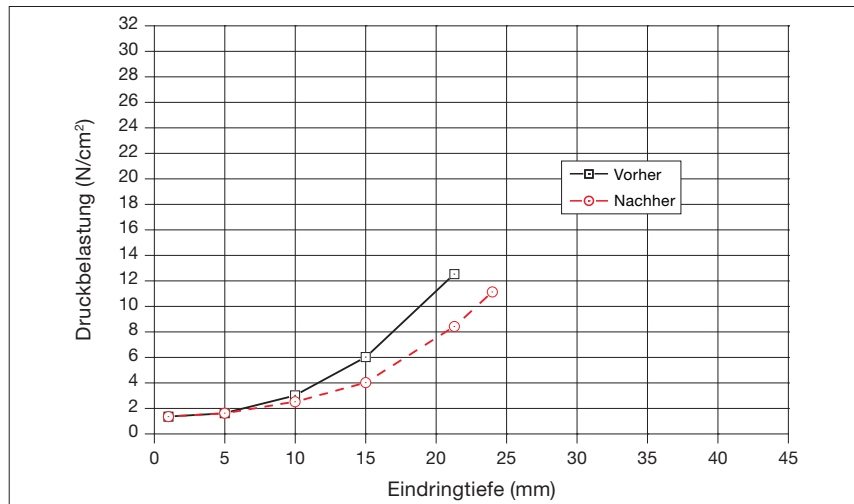
Bild 2: Verformbarkeit in Abhängigkeit vom Auflagedruck
